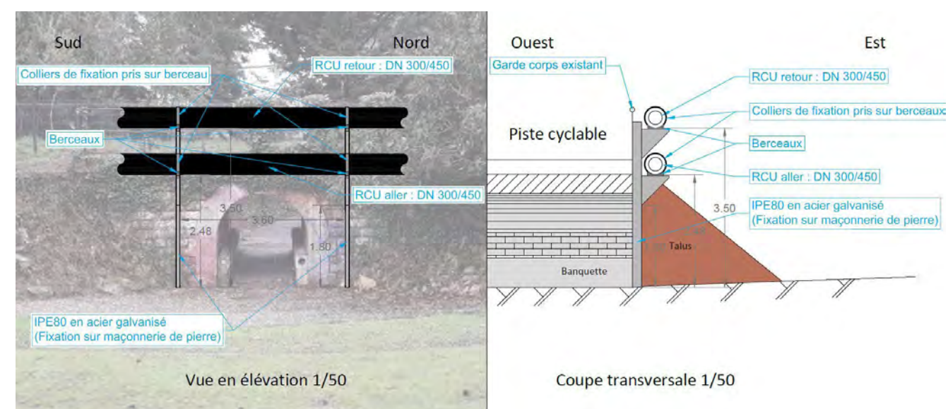
Figure 8 – Vue et coupe du Réseau de Chaleur Urbain projeté
