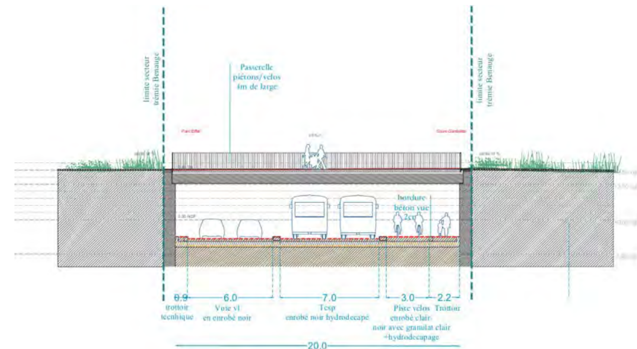
Figure 10 – Coupe en travers de la trémie Benauges
