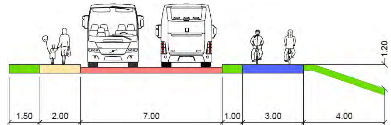
Figure 17 : Profil en travers projet – section trémie / Richelieu
