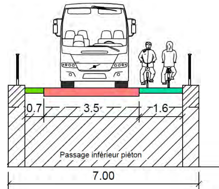
Figure 19 : Coupe en travers projet au niveau de l'ouvrage d'art existant
