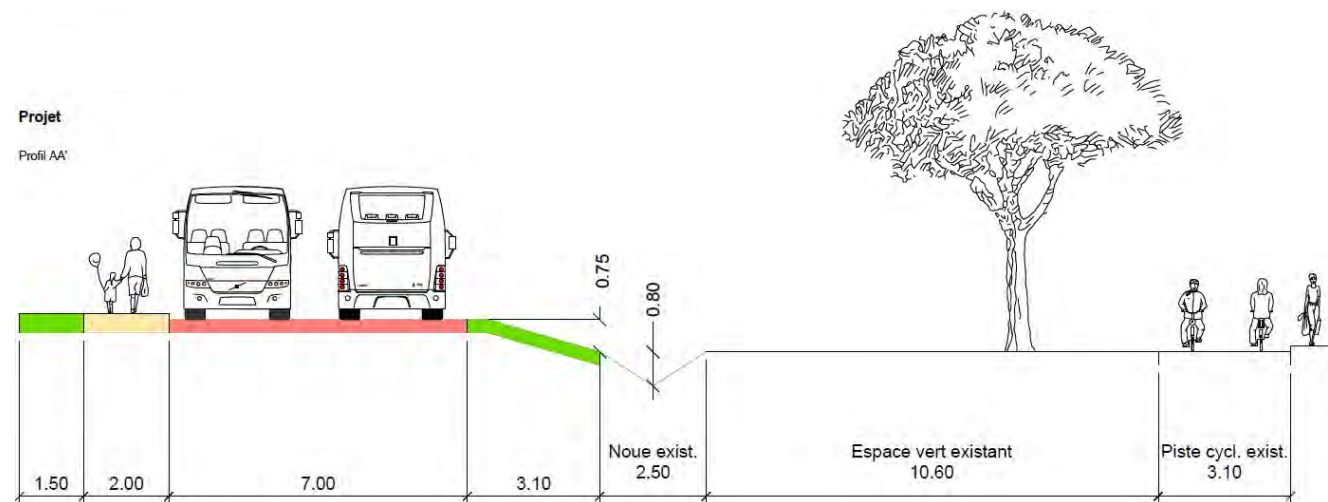
Figure 21 : Profil en travers projet – entre le chemin de Richelieu et la rue P. Laffargue
