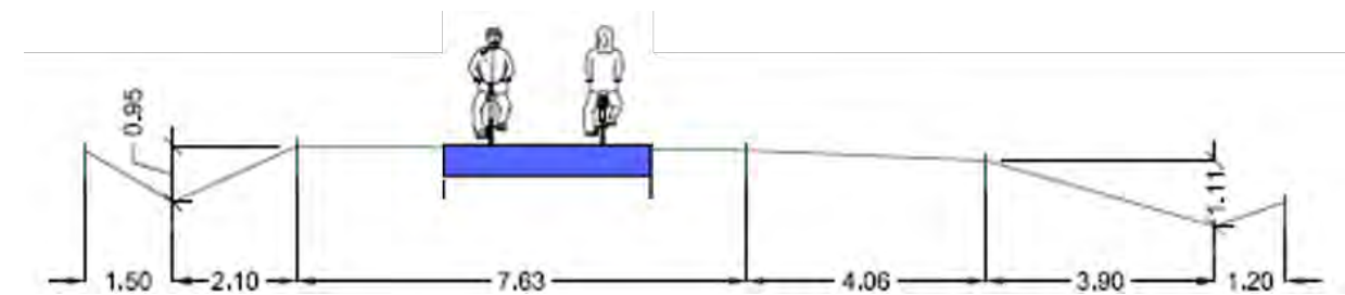
Figure 16 : Profil en travers de l'existant – section trémie / Richelieu
