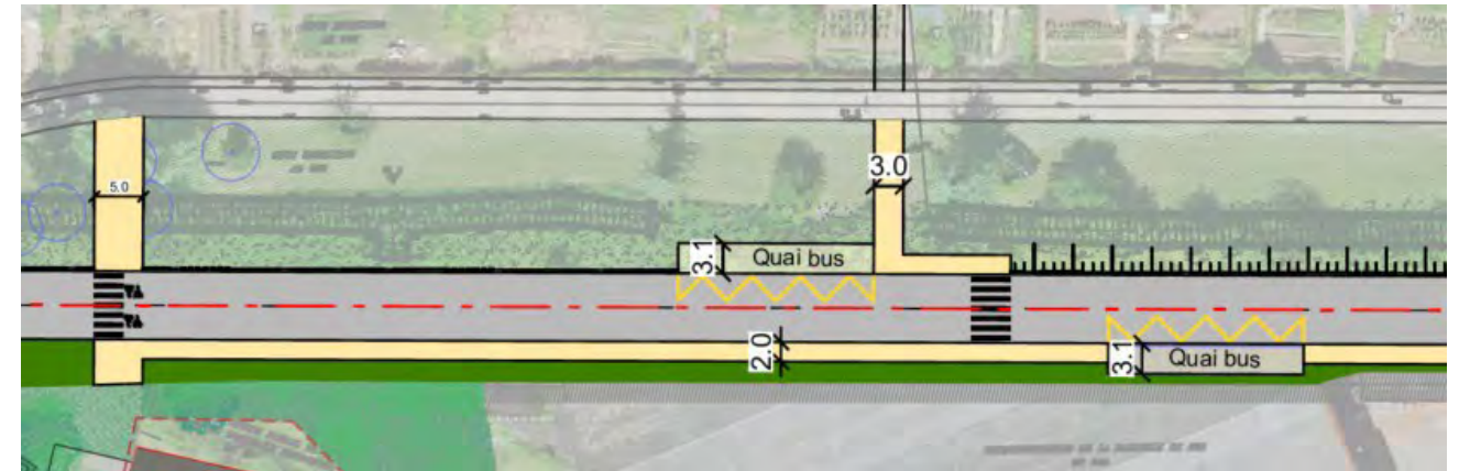
Figure 22 : Extrait des plans d'aménagement – cheminements modes doux en direction des jardins partagés
