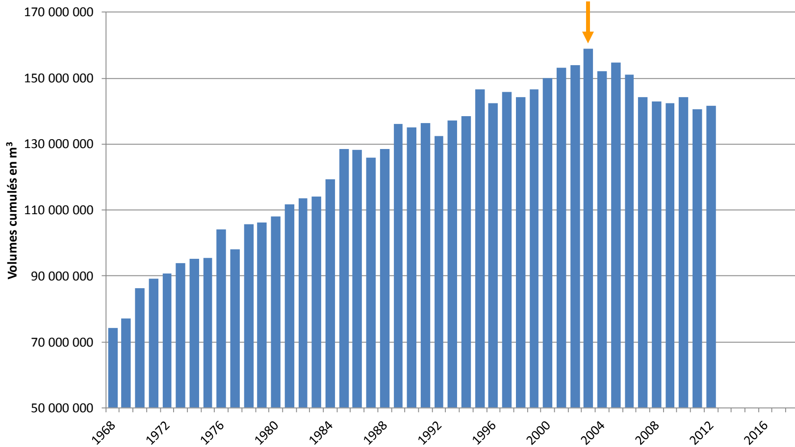
Prélèvements annuels cumulés dans les nappes profondes de Gironde
