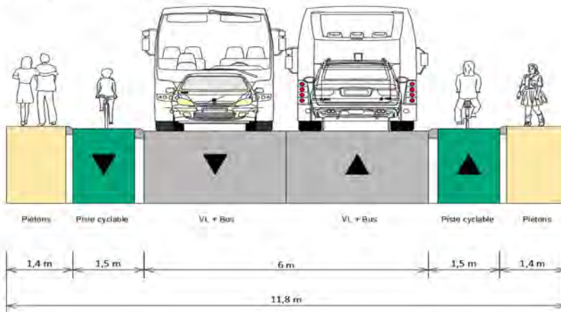
Piste cyclable à la Copenhaguoise
