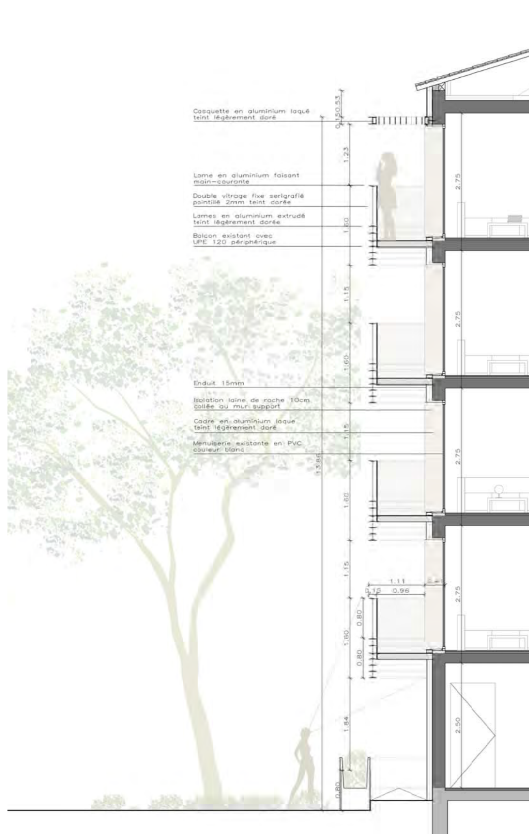
PROJET DE DENSIFICATION DE LA RESIDENCE JEAN MOULIN GIRONDE HABITAT - RCR ARTOTEC 27 MAI 2014 DETAIL DE LA FACADE DONNANT SUR L'AVENUE - RENOVATION DES BALCONS
