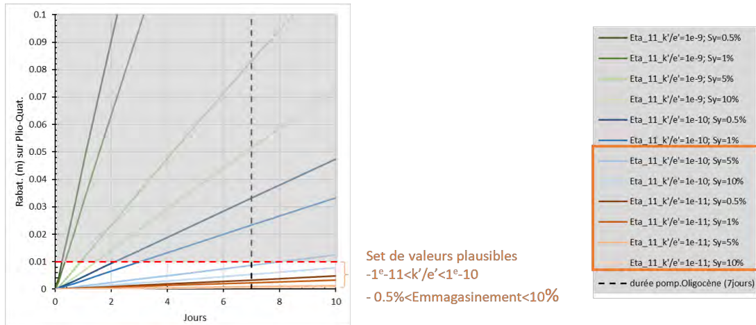
Figure 29 : Simulation de l'impact au Plio-Quaternaire lors du pompage à l'Oligocène pendant 7 jours à 200 m 3 /h
