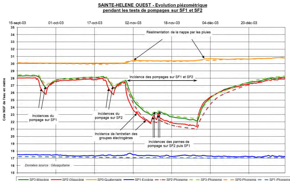
Figure 27 : Reproduction par le modèle des tests d'exploitation réalisés à grande échelle en 2003
