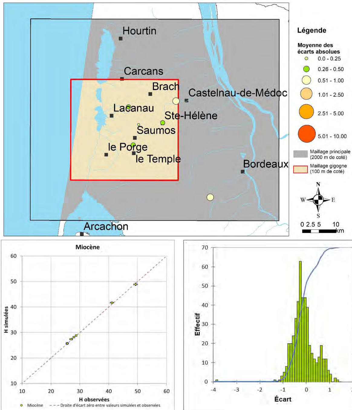
Figure 39 : Illustration des écarts de calage pour les nappes du Miocène (Aquitarien et Langhien-Serravallien)
