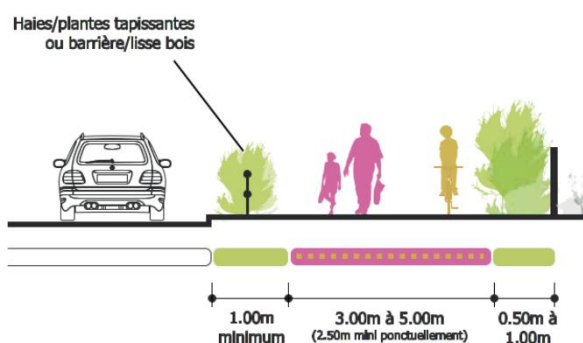
Schéma de principe d'une voie verte
