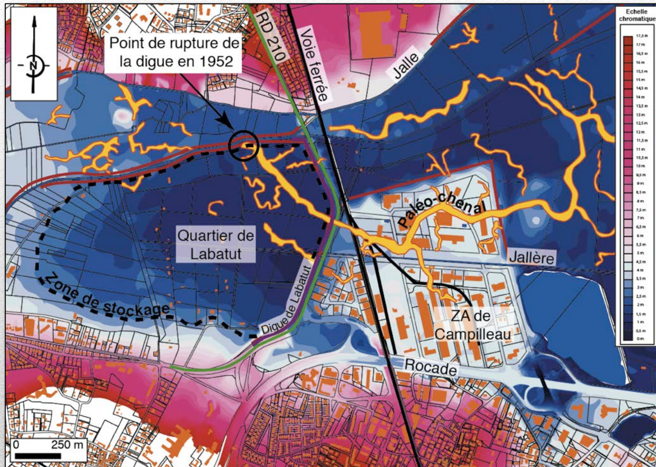
Localisation du point de rupture de la digue du Sable lors de l'inondation de 1952
