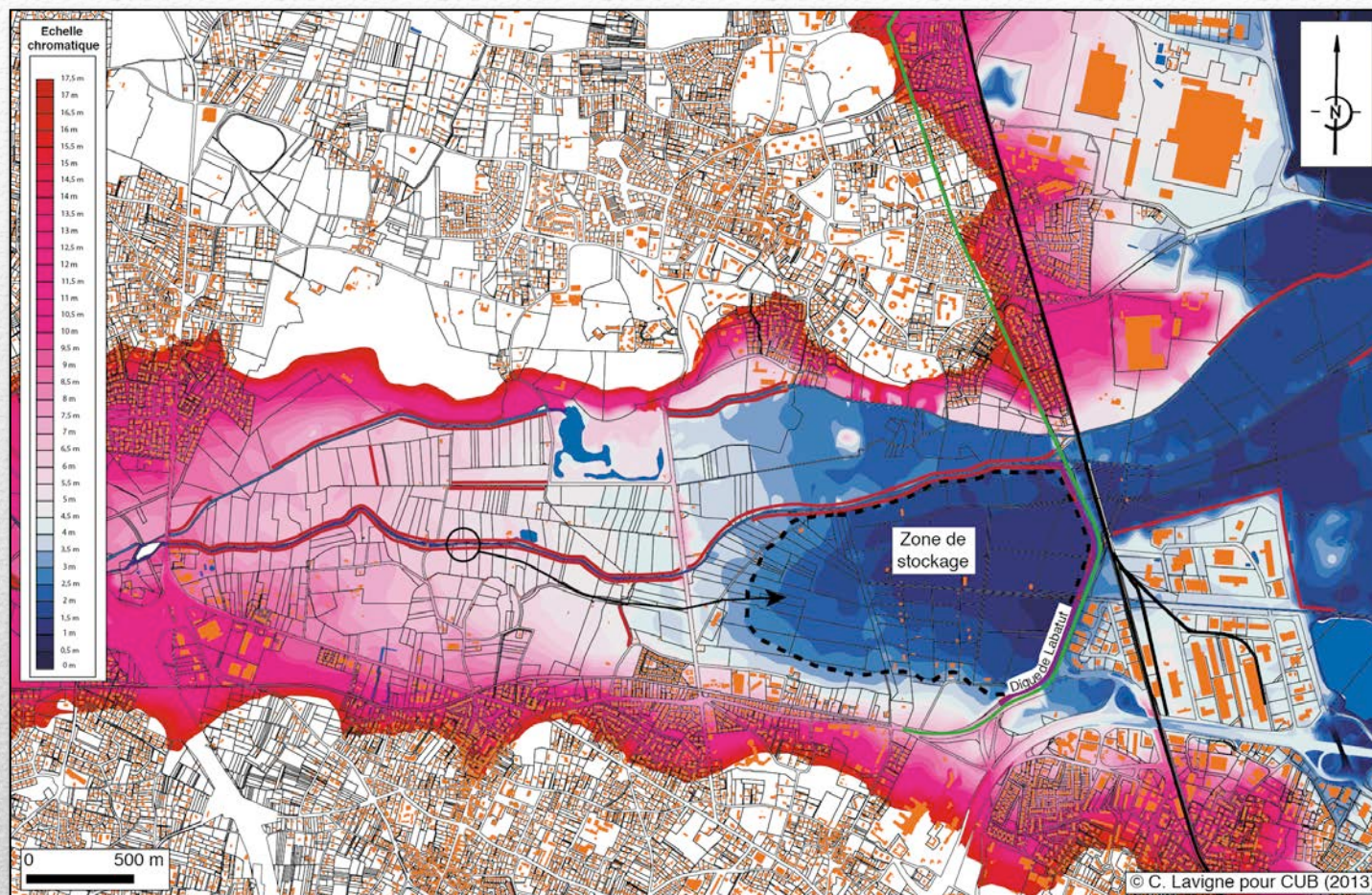
Scénario d'inondation en cas de rupture de la digue sud de la Jalle d'Eysines
